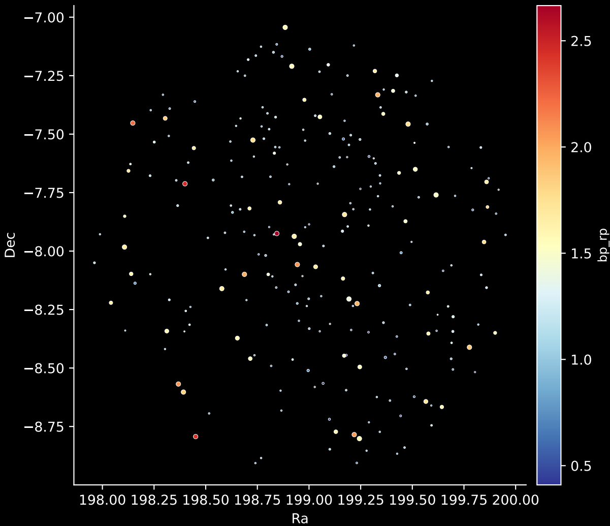
GALAH DR4 Field: [8959] Stars: 242
