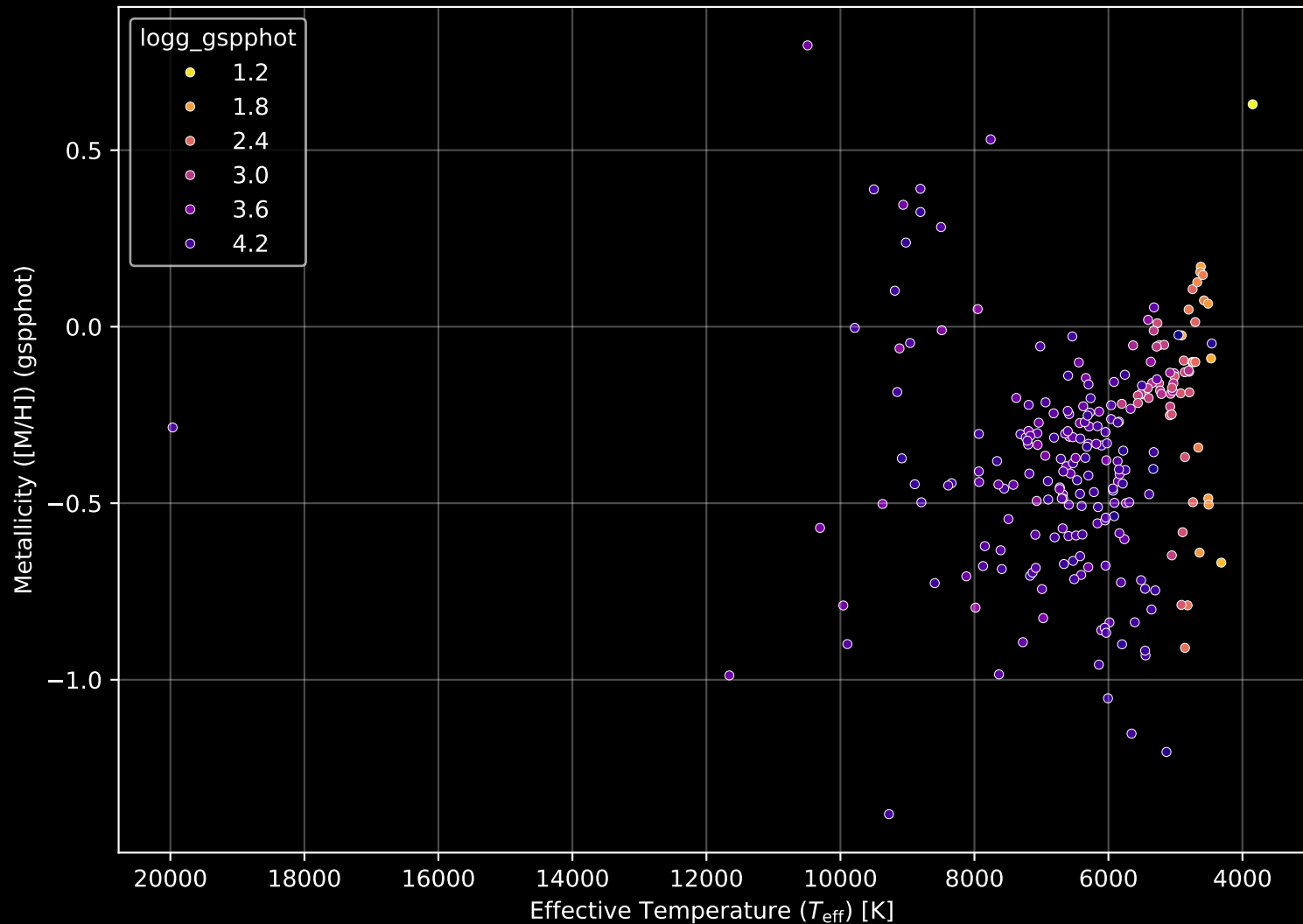
GALAH DR4 Field: [8959] Stellar Population Parameters (n= 242)
