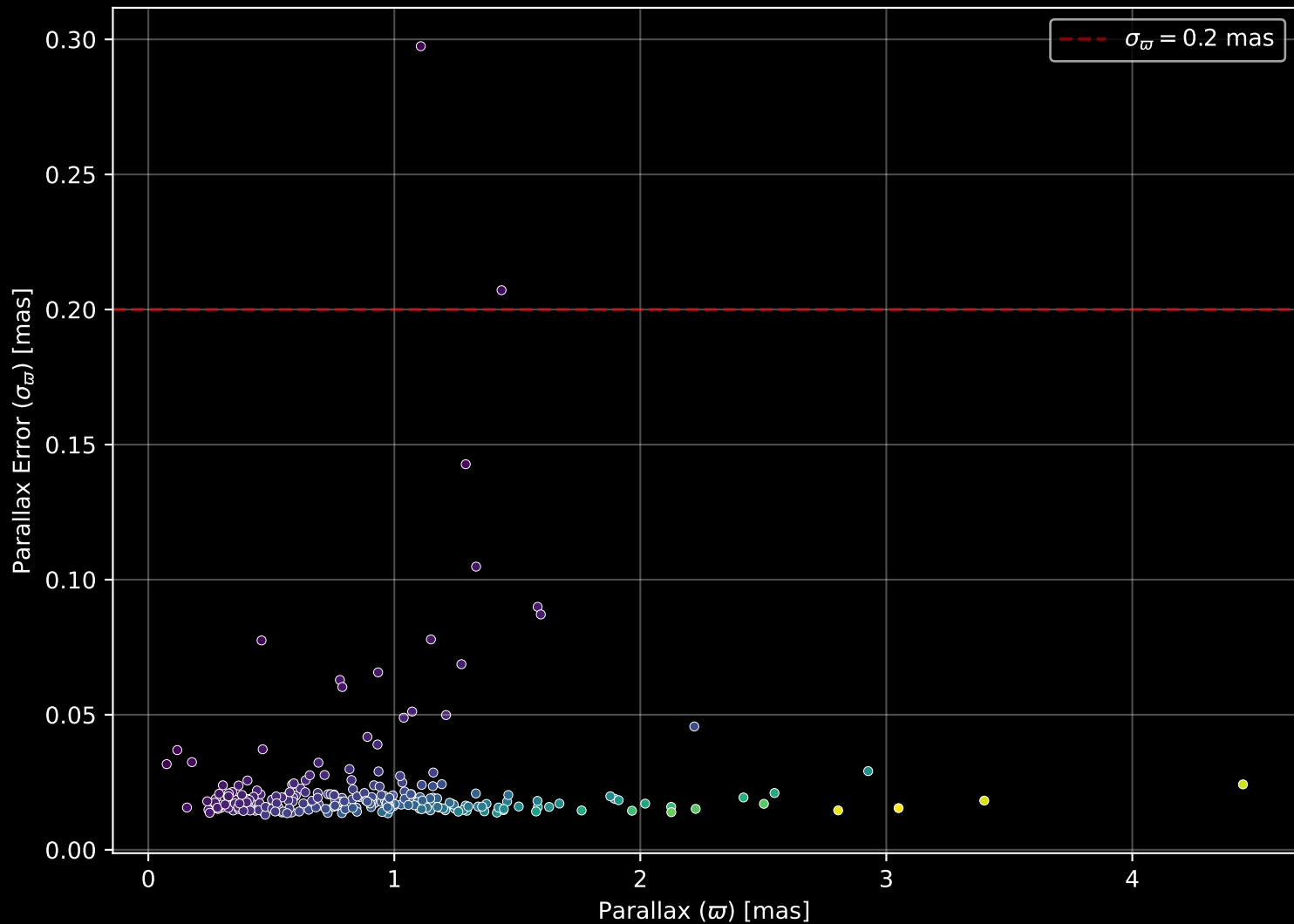
GALAH DR4 Field: [8959] Parallax Quality (n= 242)
