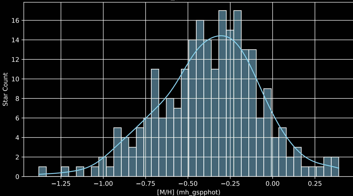
GALAH DR4 Field: [8959] [M/H] (mh_gspphot) (n= 239)
